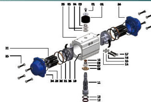
卧式执行器 Rack&Pinion Actuator
