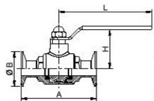
两通球阀 Straight Ball Valve DIN
